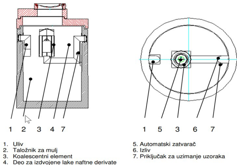
Slika 2: šematski prikaz konstrukcije separatora K NG30
